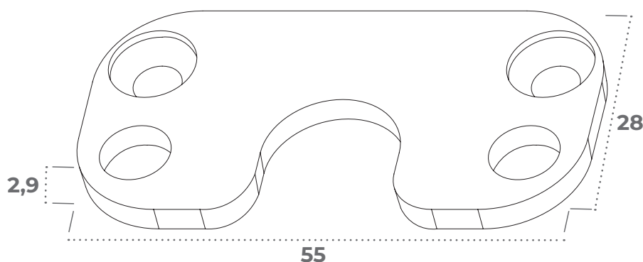
ENTRETOISE RENVOI DE FOUILLOT B552003DIIS
