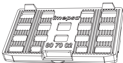
CALE DE VITRAGE MONOBLOC REHAU B807002CM1C
