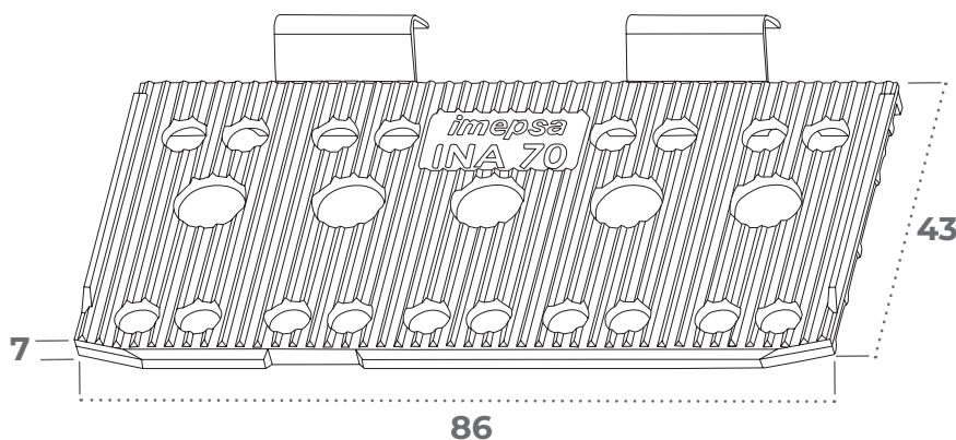
CALE DE FOND DE FEUILLURE B807015PVC
