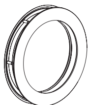
HUBLLOT MULTIPAN ROND DIA 315 CADRE EXTÉRIEUR ABA 3 mm ET CADRE INTÉRIEUR ABS PLUS DOUBLE VITRAGE 31 mm OPALE B113738931601HR5C
